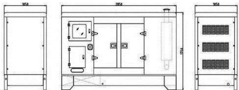
Tipo con Cabina Dimension: 2950x1100x1800mm(L*W*H) Peso: 1723kg
