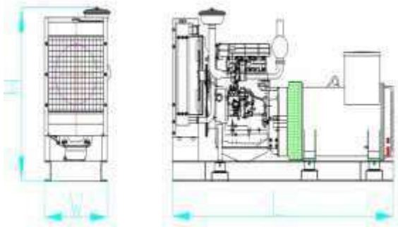
Tipo sin Cabina (Configuración Estándar) Dimension: 2144x785 x1365mm(L*W*H) Peso: 1243kg
